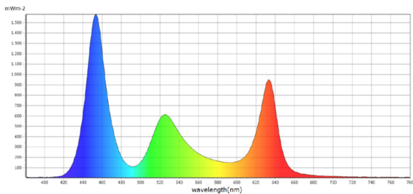
■ CIE1931
