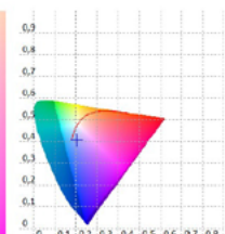
■ CIE1976
