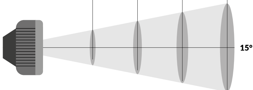
■ Spektrum
